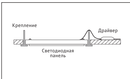
Рисунок 4. Встраиваемый монтаж в потолок типа «Армстронг»
