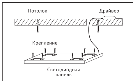
Рисунок 5. Накладной монтаж
