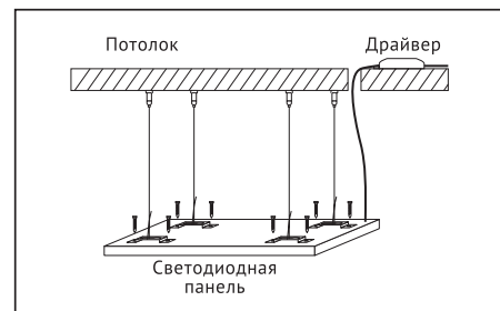
Рисунок 6. Подвесной монтаж
